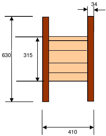
Bobina a norme ANIE 600
