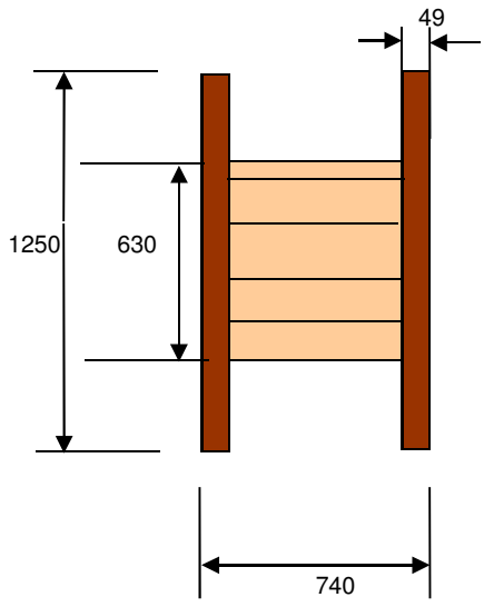
Bobina a norme ANIE 1200
