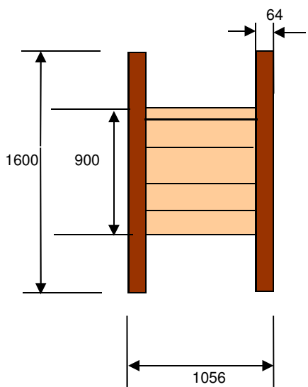
Bobina a norme ANIE 1600
