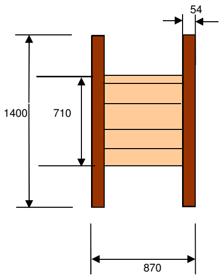
Bobina a norme ANIE 1400
