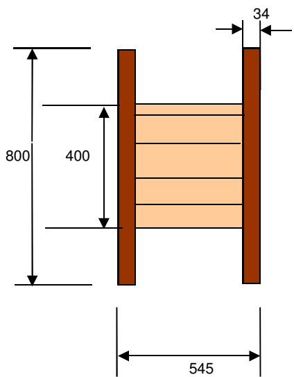
Bobina a norme ANIE 800
