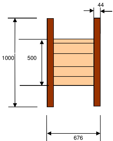
Bobina a norme ANIE 1000
